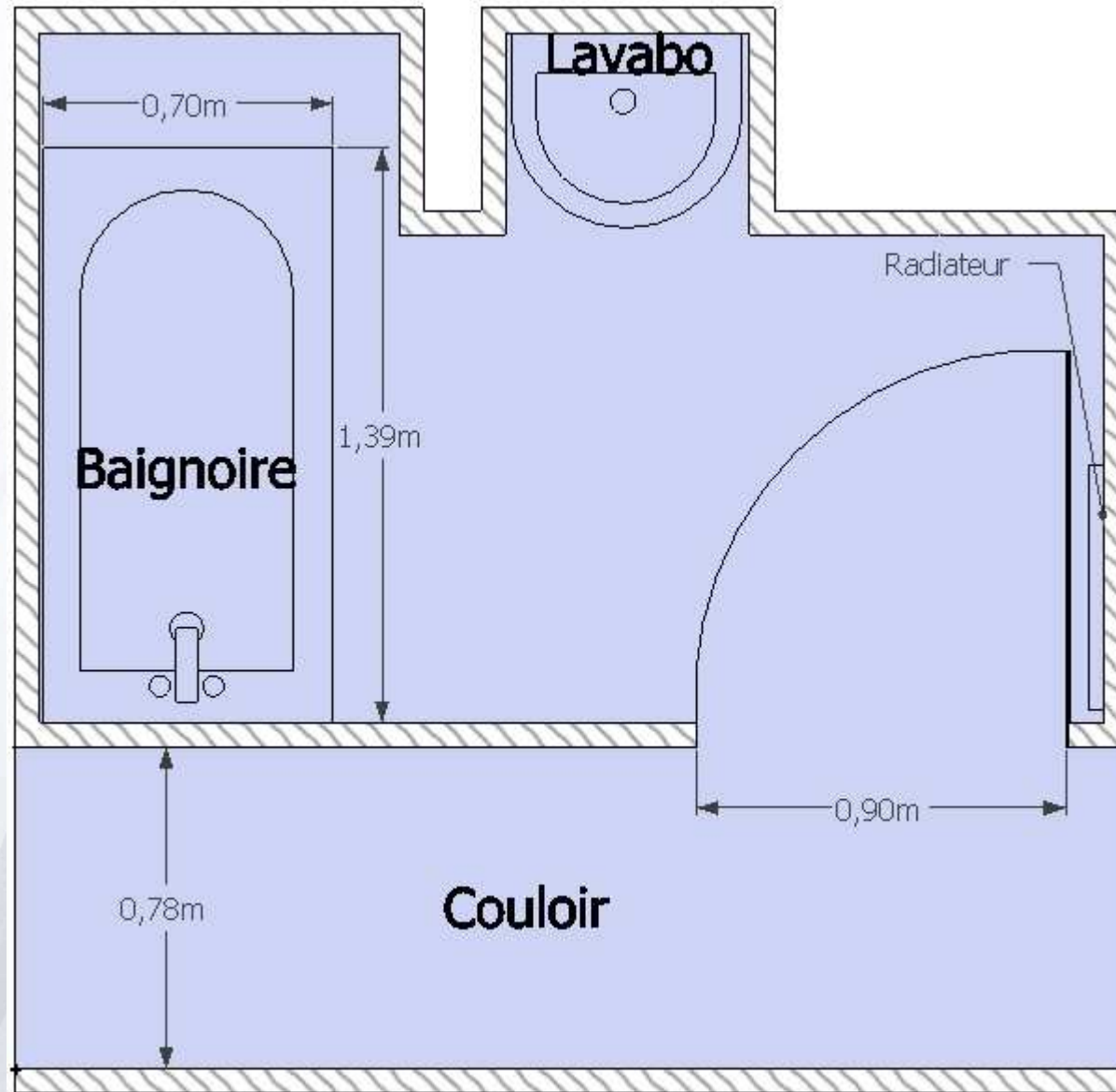
Plan de la salle de bain aménagée
